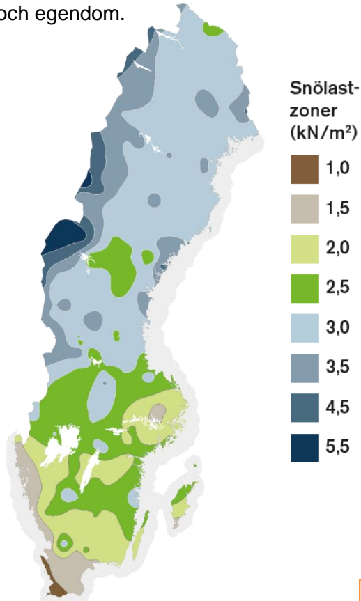
Karta för snözoner enligt EKS10 2015. Online-karta www.boverket.se , sök Snölastzoner.
